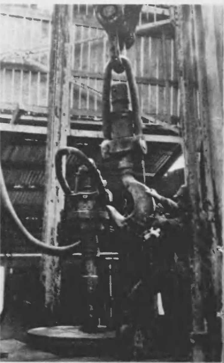
掘削作業 坑内上方から吊下つた掘管身降用の四車フックとフックの作業。左側のホースは掘泥水を循環用のロータリー・ホース。右側のホースは掘泥水をラックで製油場へ運ばれる
