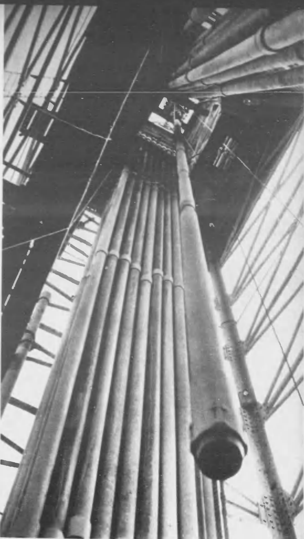
掘削の開始 この地下にはきつと油層があるぞ！四羽ビートを掘管の先端につけて、これから掘削が始まる
